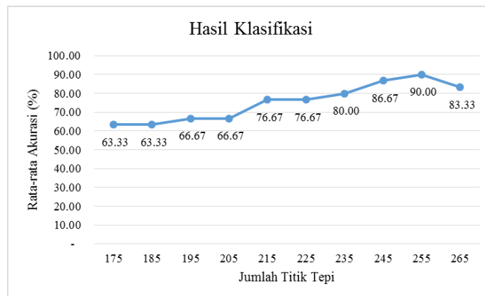
Gambar 5. Rata-rata Akurasi Bagian Kepala Ikan
